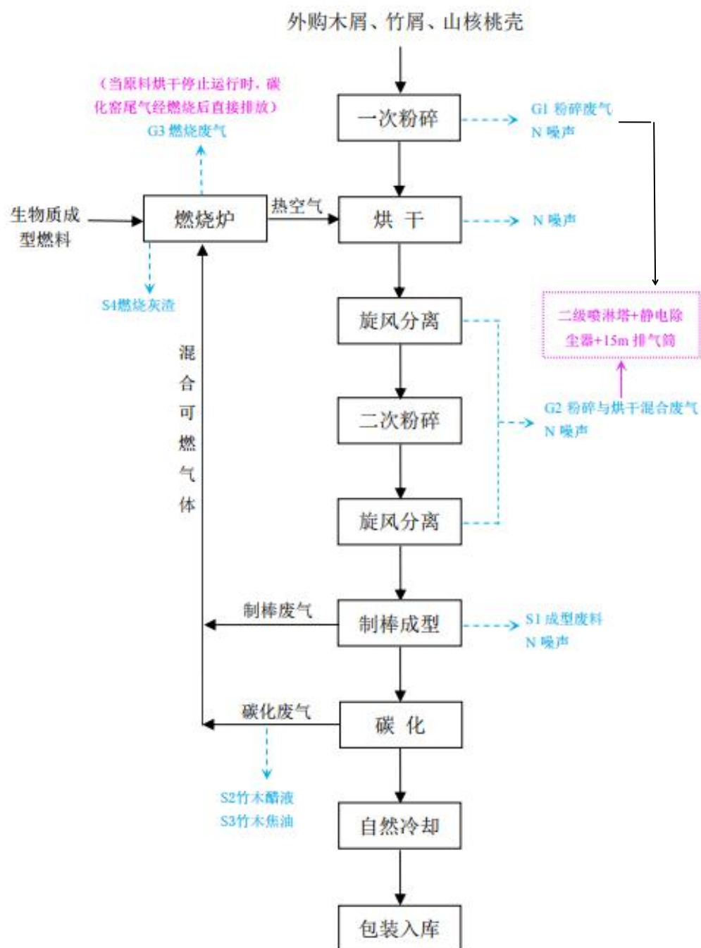
图 5-1 生产线工艺流程及产污节点图
